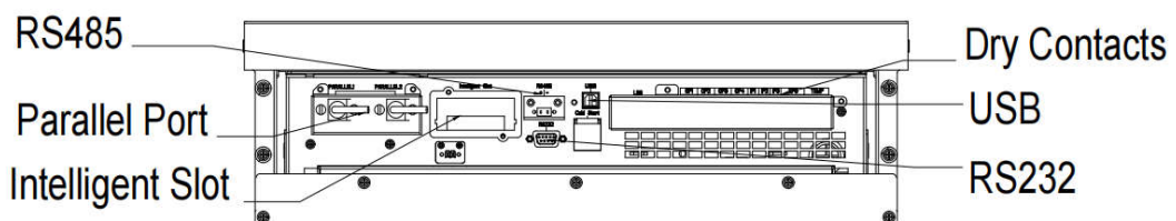
(d)10-40kVA standard backup time
